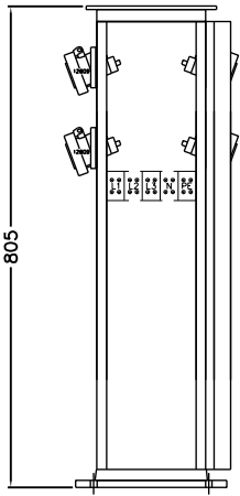
KÄYTTÖÖVI AVATTUNA
