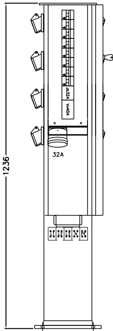
KÄYTTÖOVI AVATTUNA
